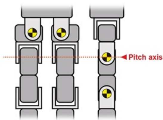
図5-3 ピッチ軸
